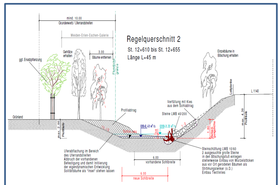
Planzustand
