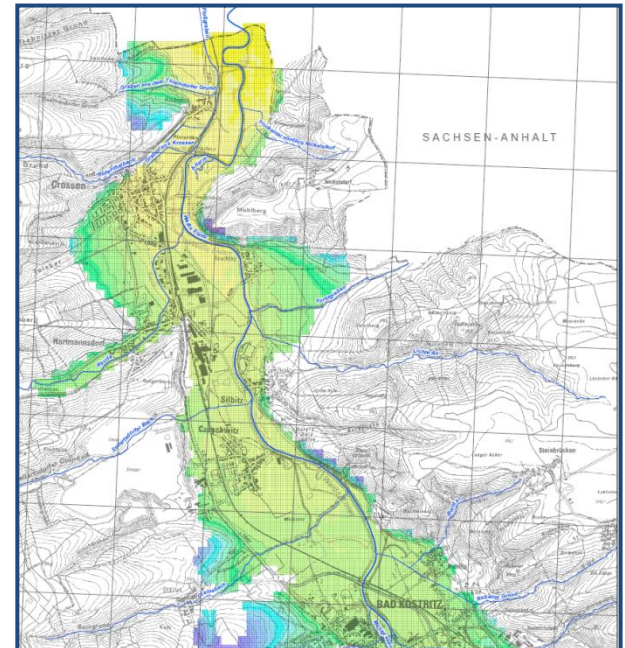
Grundwassermodell über die Talau der Weißen Elster
