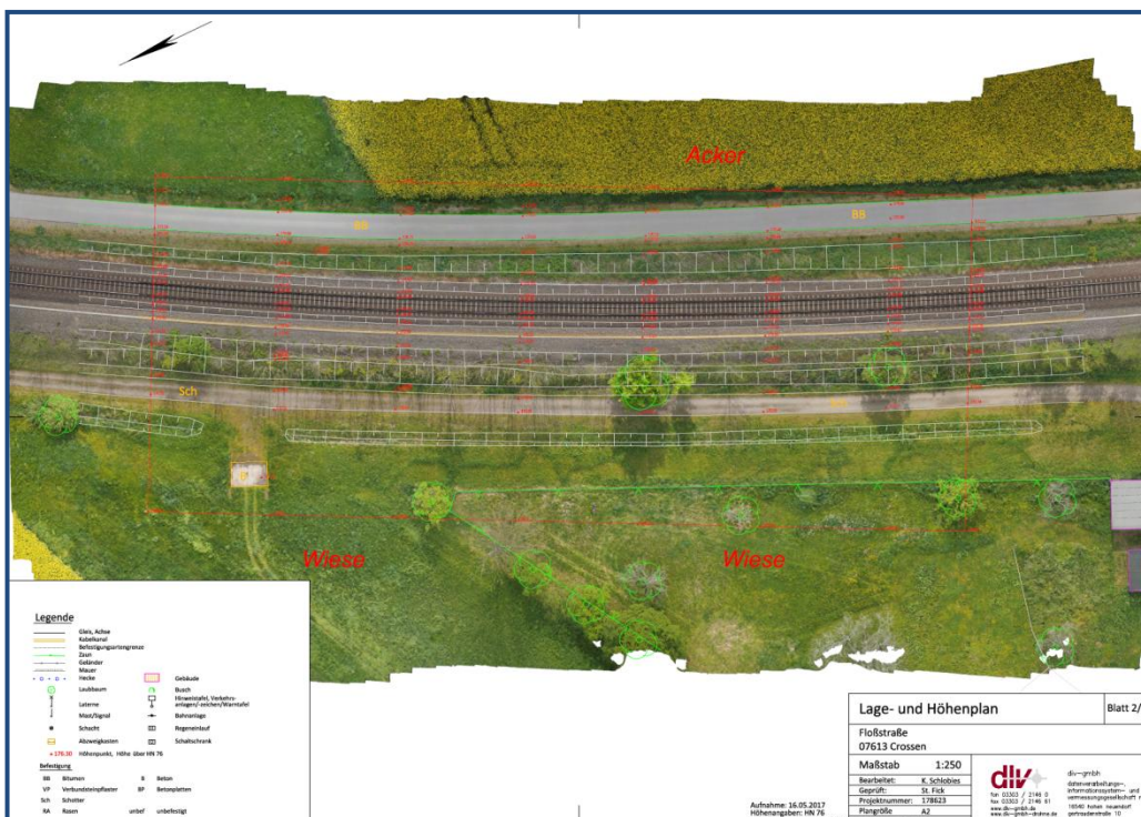
Drohngestützte Bahnvermessung mit hochauflösendem Orthofoto
