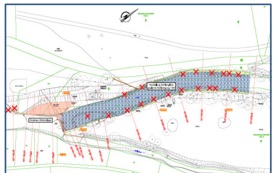
Variante 2: Sohlengleite
