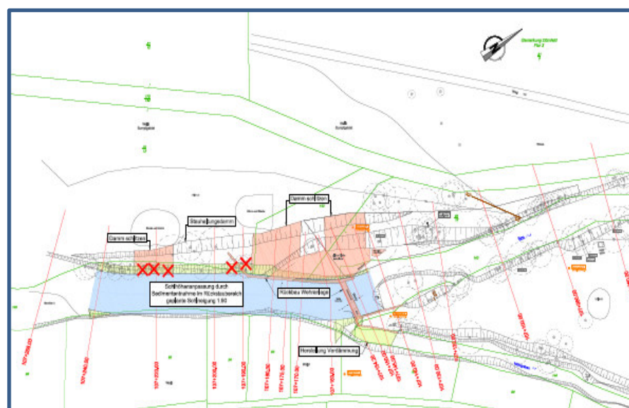
Variante 1: Rückbau
