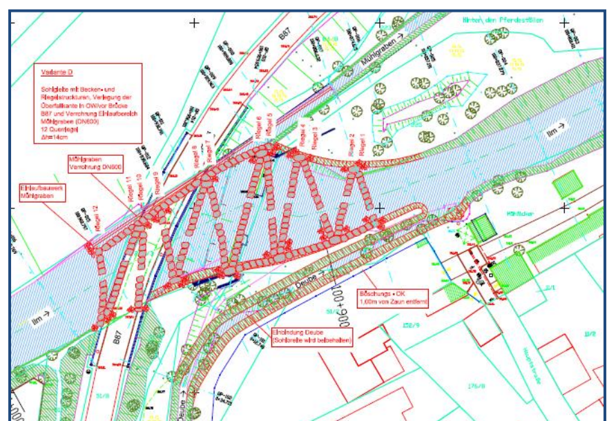
Variante 2: Sohlgleite
