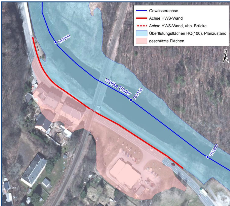
geplante Hochwasserschutzwand mit zukünftig geschütztem Areal (rot)
