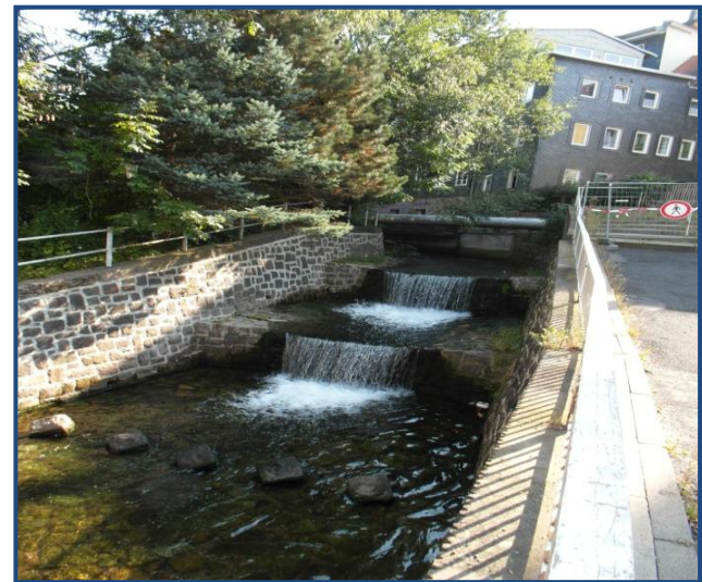
Querbauwerk LA10
