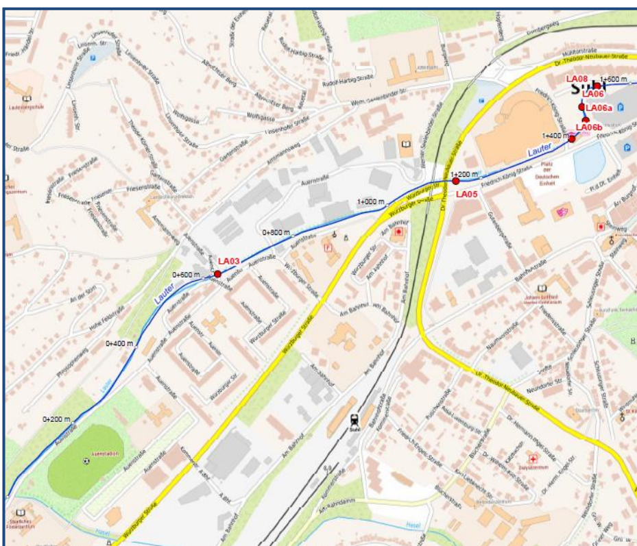
Übersichtslageplan Projektgebiet von Mündung bis Flusskilometer 1+600
