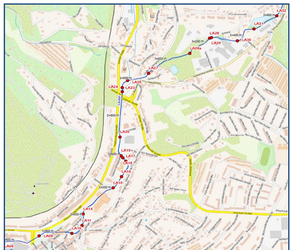
Übersichtslageplan Projektgebiet von Flusskilometer 1+600 bis Flusskilometer 3+600
